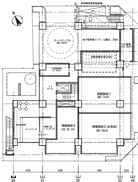
1階平面図
