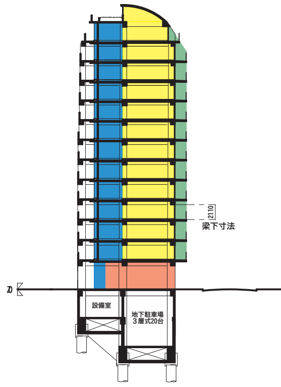
A-A断面図
